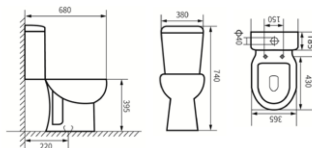
Inodoro con salida vertical
