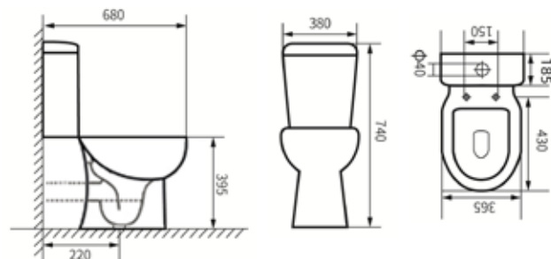
Inodoro con salida horizontal
