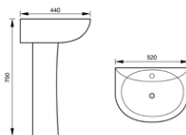
Lavabo con pedestal
